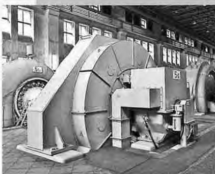
▲発電機
